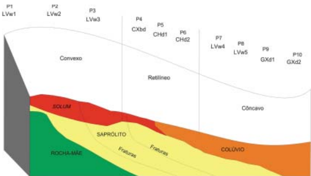
Figura 3 – Esquema da organização da pedossequência estudada neste trabalho.
